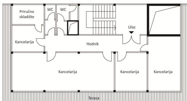
Skica poslovnog prostora
